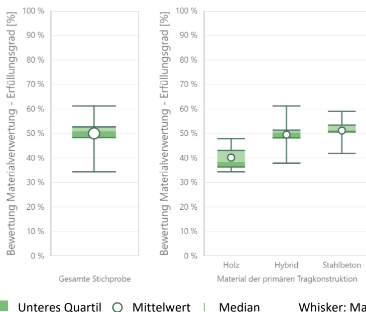
Abbildung 13: Verteilung der Daten für den Kennwert der Materialverwertung (REC), für die gesamte Stichprobe und nach Material der primären Tragkonstruktion (in %)
