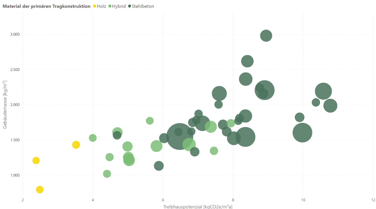
Abbildung 8: Darstellung der Stichprobe nach Masse pro NRF [kg/m 2 ] und GWP pro NRF und Jahr [kgCO 2 e/m 2 a] Farbgebung nach Material der primären Tragkonstruktion und Größe der Punkte nach NRF des Gebäudes
